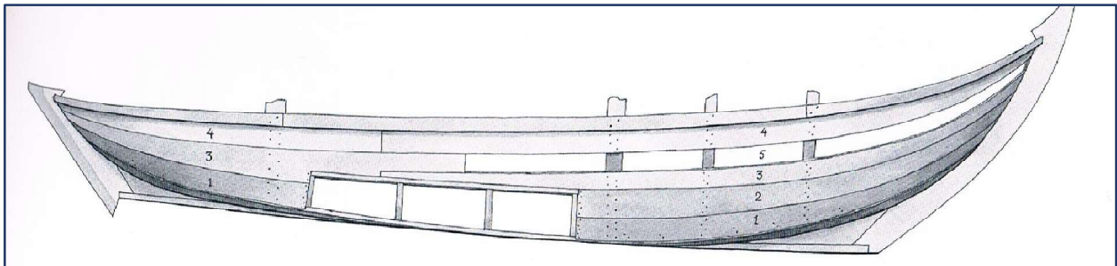
Figuur 7: Beeld van de zijkant van het schip, met haar verschillende huidgangen: 1) kimgang, 2) 2de gang, 3) lijfhoutsgang en 4) berghoutsgang (Dorleijn, 1998, p. 137).
