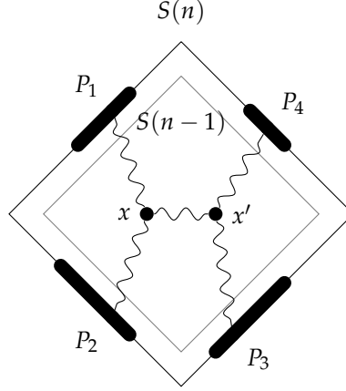
FIGUUR 4. Twee trifurcaties x, x' met corresponderende 3-partities \pi(x) = \{P_1, P_2, P_3 \cup P_4\} en \pi(x') = \{P_1 \cup P_2, P_3, P_4\} .
