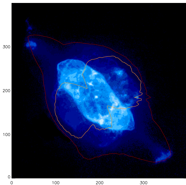
NGC 7009 (Disk)
