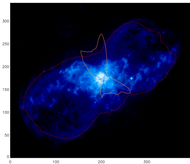
Hubble 5 (Disk)
