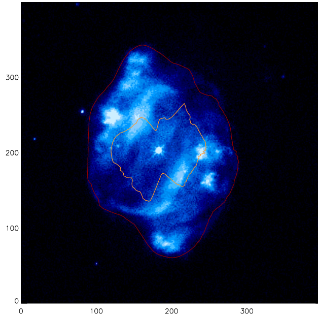
NGC 5307 (Disk)
