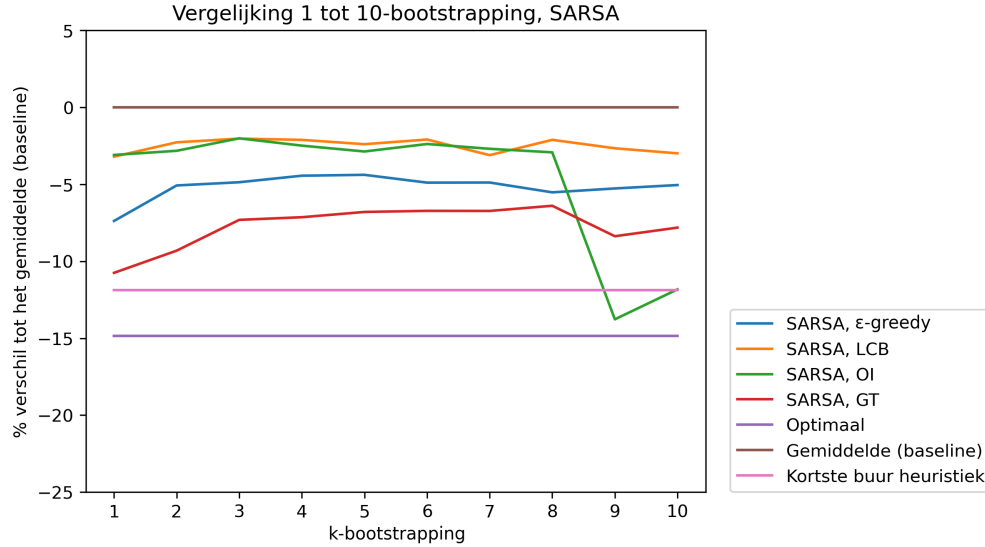
Figuur 8: k - stap -bootstrapping met on-strategie (SARSA)) algoritme met de strategieën: \epsilon -greedy, LCB, GT, OI, daarnaast de kortste buur heuristiek en de optimale oplossing voor een graaf van 10 knopen. De algoritmes worden vergeleken met de totale som van de kosten van een gemiddelde Hamiltonkring (de baseline). Omdat de algoritmes over tijd leren, wordt daar het gemiddelde genomen over de laatste 10 iteraties. De parameters die voor de on-strategie worden gekozen zijn als volgt: voor elke strategie en elke k -stap-bootstrapping van de graaf worden de volgende parameters bekeken: c, \epsilon = [0.001, 0.15, 0.3, 0.6, 0.8, 0.999] en \alpha = [0.01, 0.1, 0.3, 0.5, 0.9] . De parameters worden zo geselecteerd dat deze de laagste uitkomst geven over de laatste 10 iteraties. De grafen hebben gewichten van een uniforme verdeling. De waarden die je ziet in de grafiek zijn uit de Q tabel, die op de laatste 10 iteraties gretig worden doorlopen, startend in toestand 1 (gegeven de beste parameters).
