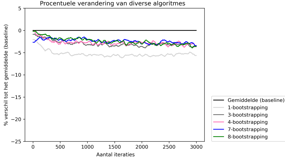
Figuur 9: k -stap-bootstrapping met off-strategie (SARSA)) algoritme met de gemiddeldes over de strategieën: \epsilon -greedy, LCB, GT, 0I, voor een graaf van 10 knopen. De algoritmes worden vergeleken met de totale som van de kosten van een gemiddelde Hamiltonkring (de baseline). We zien een leertraject over 3000 iteraties. De parameters die voor de off-strategie worden gekozen zijn als volgt, voor elke strategie en elke 1, 3, 4, 7, 8-bootstrapping van de graaf worden de volgende parameters bekeken: c, \epsilon = [0.001, 0.15, 0.3, 0.6, 0.8, 0.999] en \alpha = [0.01, 0.1, 0.3, 0.5, 0.9] . De parameters worden zo geselecteerd dat deze de laagste uitkomst geven over de laatste 10 iteraties. We bekijken voor elke 1, 3, 4, 7, 8-stap-bootstrapping van de graaf 10 grafen, waarbij de grafen gewichten hebben van een uniforme verdeling. De smoothing window = 51. De waarden die je ziet in de grafiek zijn uit de Q tabel, die op de zoveelste iteratie gretig wordt doorlopen, startend in toestand 1 (gegeven de parameters).
