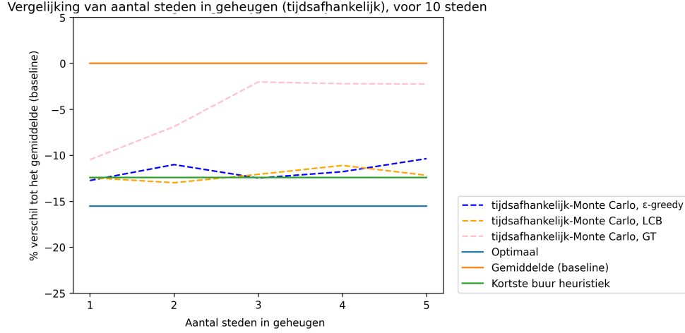
Figuur 15: Monte Carlo algoritme met de strategieën: \epsilon -greedy, LCB, GT, daarnaast de korste buur heuristiek en de optimale oplossing. De algoritmes worden vergeleken met de totale som van de kosten van een gemiddelde Hamiltonkring (de baseline). Omdat de Monte Carlo algoritmes gedurende de tijd leren, wordt het gemiddelde genomen over de laatste 10 iteraties. De parameters die voor Monte Carlo worden gekozen zijn als volgt, voor elke strategie en elke grootte van de toestandsruimte worden de volgende parameters bekeken: c, \epsilon = [0.001, 0.15, 0.3, 0.6, 0.8, 0.999] en \alpha = [0.01, 0.1, 0.3, 0.5, 0.9] . De parameters worden zo geselecteerd dat deze de laagste uitkomst geven over de laatste 10 iteraties. We bekijken voor elke grootte van de toestandsruimte 10 grafen. De grootte van de toestandsruimte wordt gevarieerd door het aantal laatst bezochte steden te variëren. De Q tabel wordt voor elke tijd T gemaakt, zodat de toestandsruimte nog groter is. Tot slot hebben de grafen gewichten van de uniforme verdeling. De waarden die je ziet in de grafiek zijn uit de Q tabel, die op de laatste 10 iteraties gretig worden doorlopen, startend in toestand 1 (gegeven de parameters).
