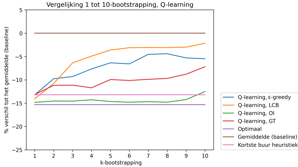
Figuur 10: k-stap-bootstrapping met on-strategie (Q-learning) algoritme met de strategieën: \epsilon -greedy, LCB, GT, OI, daarnaast de kortstebuur heuristiek en de optimale oplossing voor een graaf van 10 knopen. De algoritmes worden vergeleken met de totale som van de kosten van een gemiddelde Hamiltonkring (de baseline). Omdat de on-strategie algoritmes over tijd leren, wordt daar het gemiddelde genomen over de laatste 10 iteraties. De parameters die voor de on-strategie worden gekozen zijn als volgt: voor elke strategie en elke k -bootstrapping van de graaf worden de volgende parameters bekeken: c, \epsilon = [0.001, 0.15, 0.3, 0.6, 0.8, 0.999] en \alpha = [0.01, 0.1, 0.3, 0.5, 0.9] . De parameters worden zo geselecteerd dat deze de laagste uitkomst geven over de laatste 10 iteraties. We bekijken voor elke k -stap-bootstrapping van de graaf 10 grafen, waarbij de grafen gewichten hebben van een uniforme verdeling. De waardes die je ziet in de grafiek zijn uit de Q tabel, die op de laatste 10 iteraties gretig worden doorlopen, startend in toestand 1 (gegeven de beste parameters).
