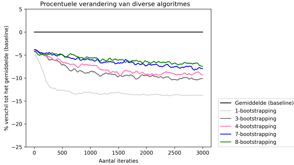
Figuur 11: k-stap-bootstrapping met on-strategie (Q-learning) algoritme met de gemiddeldes over de strategieën: \epsilon -greedy, LCB, GT, OI, voor een graaf van 10 knopen. De algoritmes worden vergeleken met de totale som van de kosten van een gemiddelde Hamiltonkring (de baseline). We zien een leertraject over 3000 iteraties. De parameters die voor de off-strategie worden gekozen zijn als volgt: voor elke strategie en elke 1, 3, 4, 7, 8-stap-bootstrapping van de graaf worden de volgende parameters bekeken: c, \epsilon = [0.001, 0.15, 0.3, 0.6, 0.8, 0.999] en \alpha = [0.01, 0.1, 0.3, 0.5, 0.9] . De parameters worden zo geselecteerd dat deze de laagste uitkomst geven over de laatste 10 iteraties. We bekijken voor elke 1, 3, 4, 7, 8-stap-bootstrapping van de graaf 10 grafen, waarbij de graaf gewichten hebben van een uniforme verdeling. De smoothing window = 51. De waarden die je ziet in de grafiek zijn uit de Q tabel, die op de zoveelste iteratie gretig wordt doorlopen, startend in toestand 1 (gegeven de parameters).
