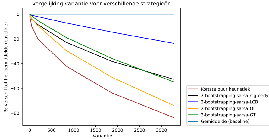
Figuur 16: 2-step-bootstrapping met on-strategie (SARSA) algoritme met de strategieën: \epsilon -greedy, LCB, GT, OI, daarnaast de kortstebuur heuristiek voor een graaf van 10 knopen, met verschillende initialisaties voor de gewichten van de takken om de grootte van de variantie te variëren. De algoritmes worden vergeleken met de totale som van de kosten van een gemiddelde Hamiltonkring (de baseline). Omdat de algoritmes over tijd leren, wordt daar het gemiddelde genomen over de laatste 10 iteraties. De parameters die voor on-strategie worden gekozen zijn als volgt, voor elke strategie en elke k -step-bootstrapping van de graaf worden de volgende parameters bekeken: c, \epsilon = [0.001, 0.15, 0.3, 0.6, 0.8, 0.999] en \alpha = [0.01, 0.1, 0.3, 0.5, 0.9] . De parameters worden zo geselecteerd dat deze de laagste uitkomst geven over de laatste 10 iteraties. We bekijken voor elke grootte van de variantie 2-bootstrapping van de graaf 10 grafen, waarbij de graaf gewichten hebben van een uniforme verdeling afhankelijk van de grootte van de variantie. De waarden die je ziet in de grafiek zijn uit de Q tabel, die op de laatste 10 iteraties gretig worden doorlopen, startend in toestand 1 (gegeven de beste parameters).
