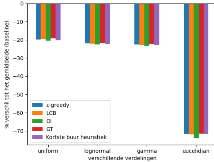
Figuur 13: 1-bootstrapping met off-strategie (Q-learning) algoritme met de strategieën: \epsilon -greedy, LCB, GT, OI, daarnaast de korste buur heuristiek voor een graaf van 50 knopen, waarbij we verschillende initialisaties van de grafen zien voor de gewichten, namelijk: Uniform, Lognormaal, Gamma, euclidisch. De algoritmes worden vergeleken met de totale som van de kosten van een gemiddelde Hamiltonkring (de baseline). Omdat de off-strategie algoritmes over tijd leren, wordt daar het gemiddelde genomen over de laatste 10 iteraties, waarbij voor 1000 iteraties geleerd wordt. De parameters die voor de off-strategie worden gekozen zijn als volgt: voor elke strategie en elke type verdeling van de gewichten en van de graaf worden de volgende parameters bekeken: c, \epsilon = [0.001, 0.15, 0.3, 0.6, 0.8, 0.999] en \alpha = [0.01, 0.1, 0.3, 0.5, 0.9] . De parameters worden zo geselecteerd dat deze de laagste uitkomst geven over de laatste 10 iteraties. We bekijken voor elke verdeling van de graaf 10 grafen (we nemen het gemiddelde van de 10 grafen), waarbij de grafen gewichten hebben van de uniforme verdeling. De waardes die je ziet in de grafiek zijn uit de Q tabel, die op de laatste 10 iteraties gretig worden doorlopen, startend in toestand 1 (gegeven de beste parameters).
