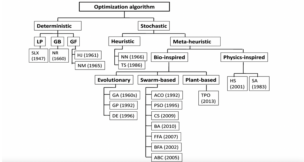
Figuur 4: Bron : zie (8). In bovenstaande afbeelding zijn verschillende oplossingsmethodes om (lokale) optima te vinden. Hierbij wordt een onderscheid gemaakt tussen stochastische en deterministische algoritmes. Bovenstaande methodes/algoritmes kunnen gebruikt worden om het HRP op te lossen.
