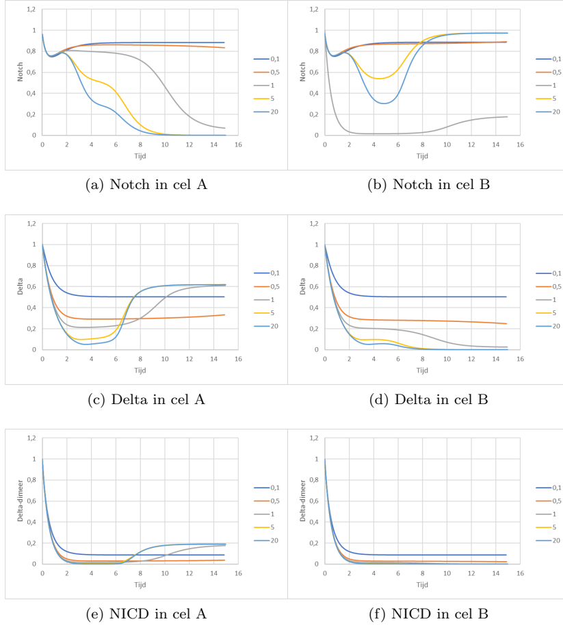
Figuur 9: Invloed van transactivatie constante \beta op het systeem met di-cis-inhibitie met vorming van dimeeren. (Vergelijkingen 18 t/m 21)
