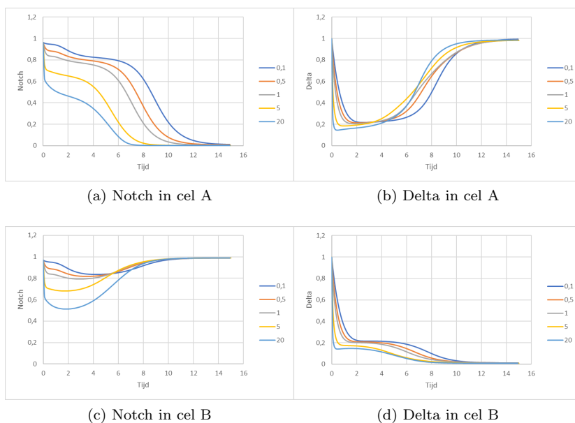
Figuur 5: Invloed van cis-inhibitie constante \alpha op het systeem met di-cis-inhibitie zonder vorming van dimere. (Vergelijkingen 22, 23 en 24)
