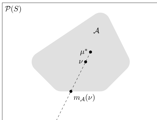
Figuur 6.1: Visualisatie van m_{\mathcal{A}}(\nu) voor een zekere \nu \in \mathcal{A} . De stippelijijn stelt de verzameling \mathcal{P}(S) \cap \{\mu^* + r(\nu - \mu^*) : r \geq 0\} voor.
