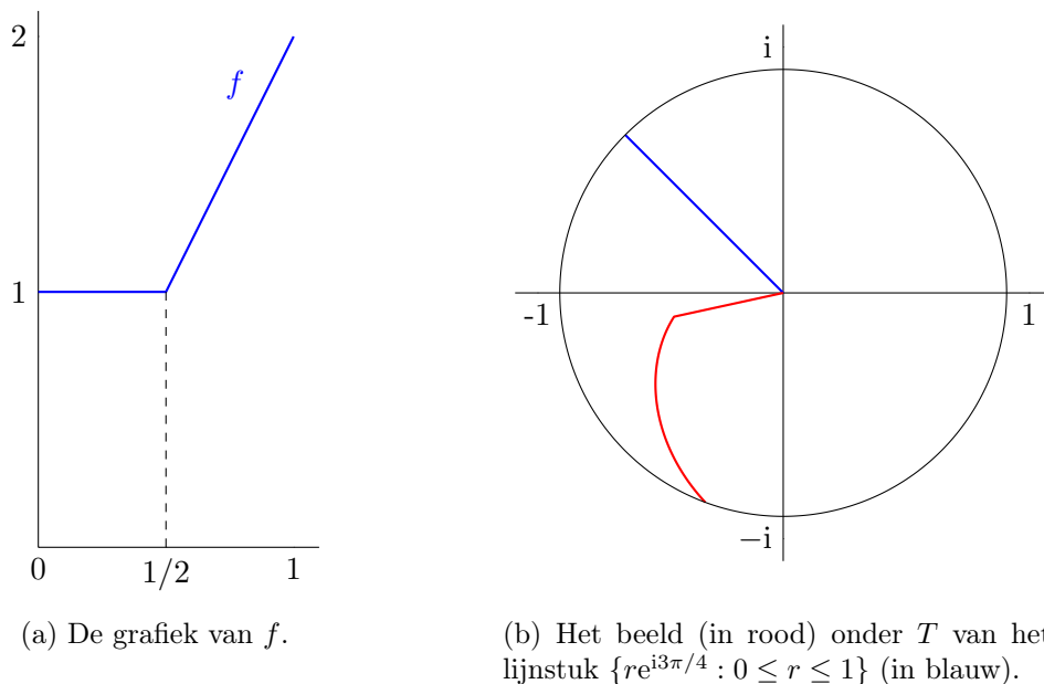
Figuur 7.1: Visualisatie van de afbeeldingen f en T uit Voorbeeld 7.2.17.
